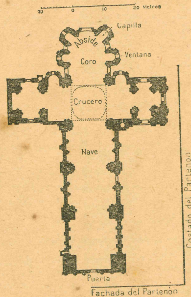
PLANO DE UNA IGLESIA ROMÁNICA. Catedral de Angulema.
