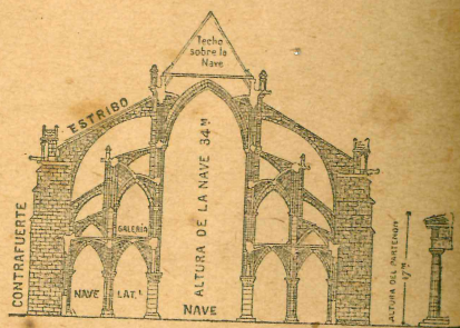
CORTE DE UNA IGLESIA OJIVAL. La catedral de París.
